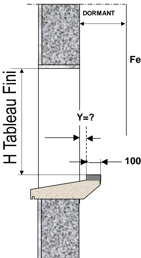
COUPE VERTICALE
