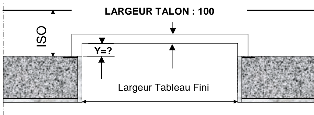
COUPE HORIZONTALE
